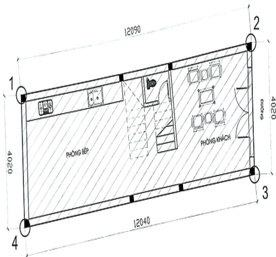
MẶT BẰNG ĐỊNH VỊ CÔNG TRÌNH
